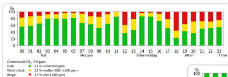
Figur 1: CO2 niveauet 'Den Gamle del', 2020
