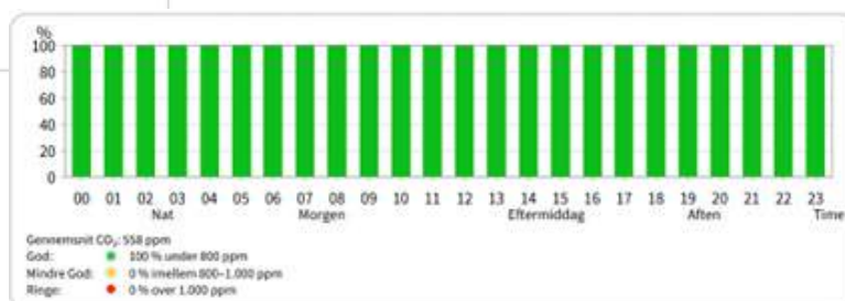
Figur 2: CO2 niveauet i den nye spisesal 2024
